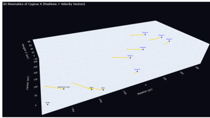
FIGURE 9 – Visualisation des objets du Cygne en 3D, centré sur le groupe E. Les lignes jaunes représentent les vecteurs vitesses
