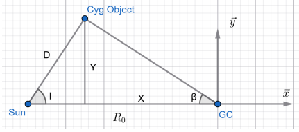
FIGURE 2 – Géométrie de projection dans le plan galactique (X, Y) .
