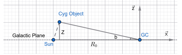
FIGURE 3 – Géométrie de projection selon l'axe vertical (Z) .
